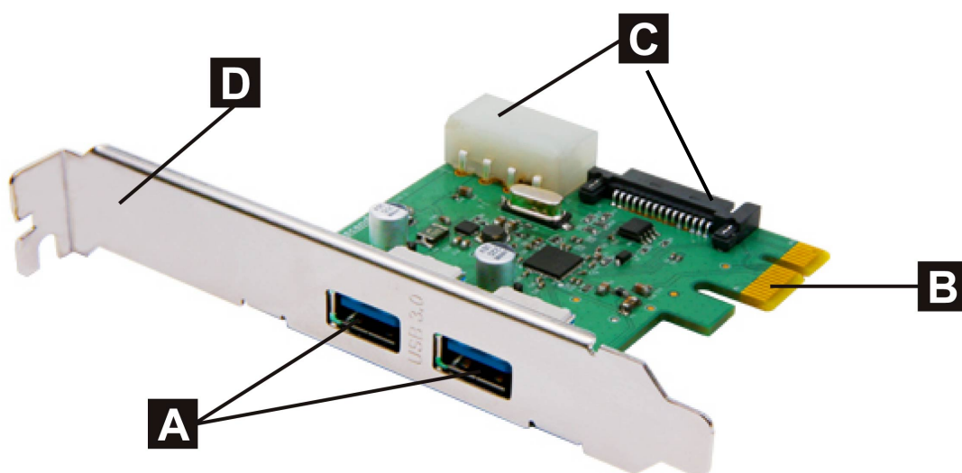
Рисунок 1: Плата расширения USB 3.0
